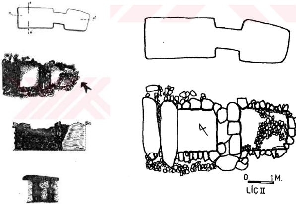
Figür 2a-b: Liç I-II Nolu Mezar Odası
