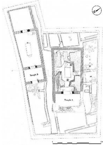
Görsel 2: Prinias A Tapınağı Planı.
