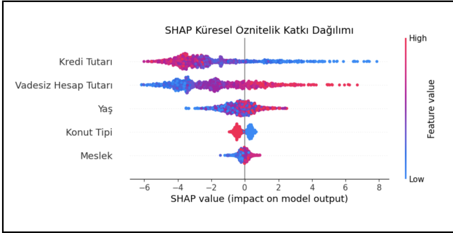
Resim 4 : SHAP arı sürüsü (beeswarm) görselleştirme: Öznitelik katkılarının veri kümesi boyunca dağılımı
