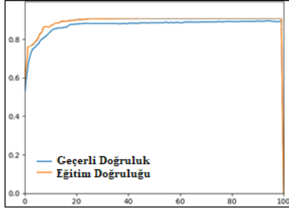
Şekil 5. EKG verisini özellik olarak kullanan ESA mimarisinin doğruluğu
