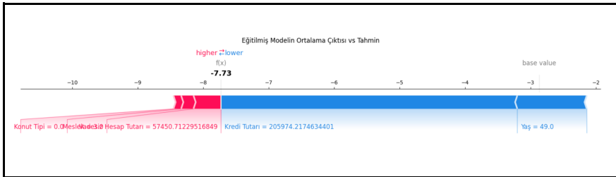
Resim 5 : SHAP güç (force) grafiği görselleştirmesi
