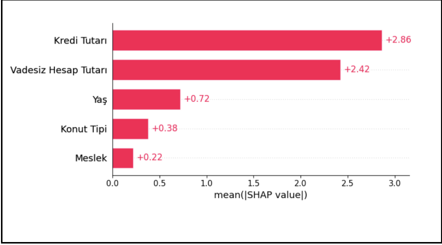
Resim 3 :SHAP özet grafiği :Özniteliklerin model çıktısı üzerindeki ortalama etkileri.
