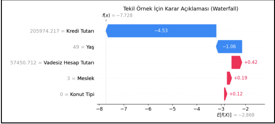
Resim 6 : SHAP şelale (waterfall) grafiği görselleştirmesi
