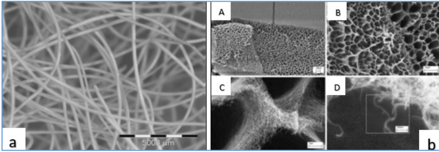
Şekil 5: Kuru yoğunluğu 124 kg/m 3 olan, süper kritik kurutmadan sonra selüloz aerogel filamentinin ışık mikroskopik resmi (a), ağırlıkça %3 selüloz içeren bir aerogel filamentinin farklı büyütmelerde SEM resmi (b)
