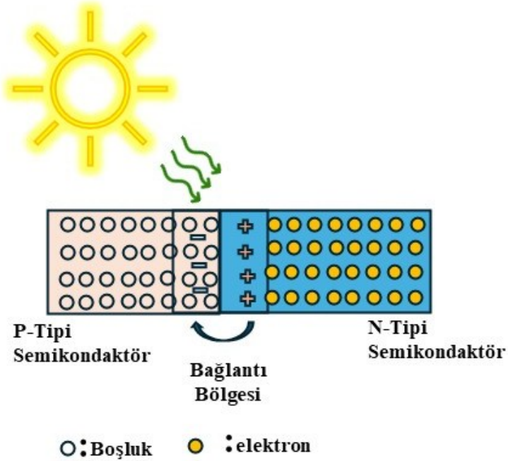
Şekil 1. Fotovolteliklerin Çalışma Prensibi Özeti
