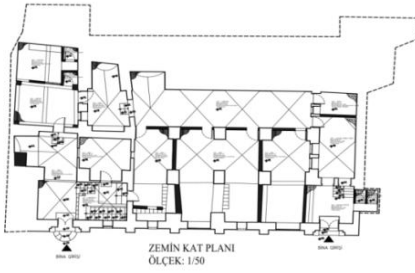
Şekil 5. Rölöve Projesi (Zemin ve 1 Kat Planı 2000)
