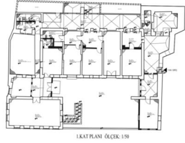
Şekil 5. Rölöve Projesi (Zemin ve 1 Kat Planı 2009)
