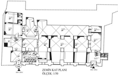
Şekil 5. Rölöve Projesi (Zemin ve 1 Kat Planı 2009)
