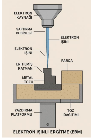
Resim 7 Elektron Işınlı Ergitme Teknolojisine Sahip 3D Yazıcı
