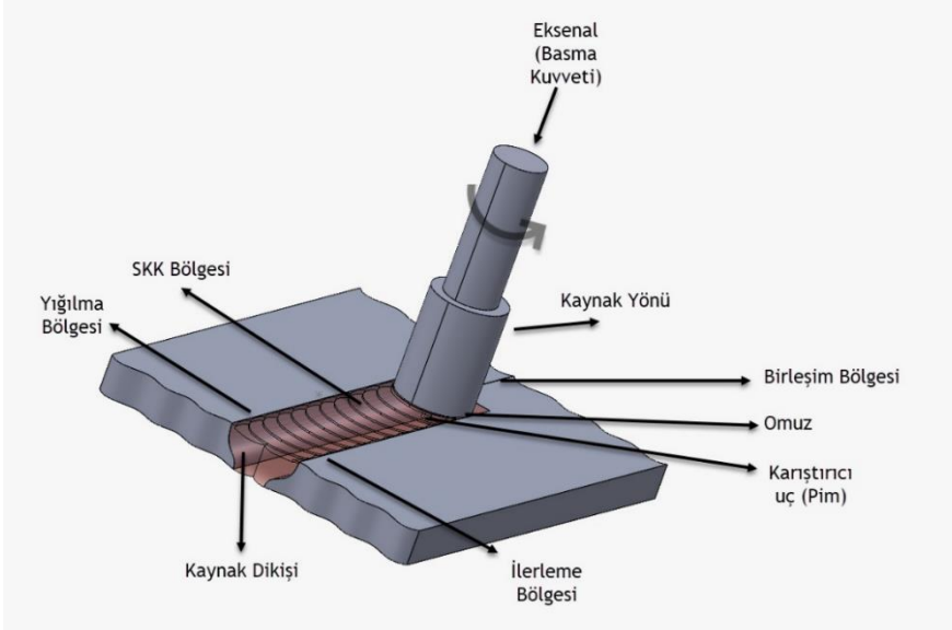
Şekil 4. Sürtünme karıştırma kaynak yönteminin şematik resmi
