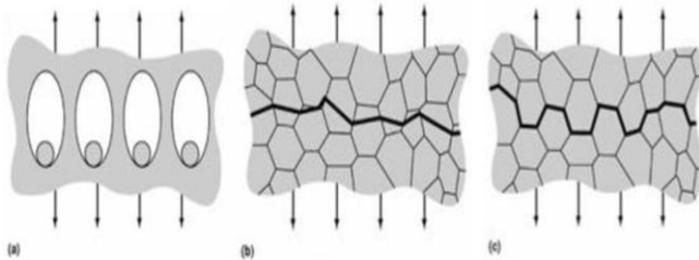
Şekil 1. Mikro boşlukların birleşmesiyle çatlağın ilerlemesi (a), Ayrılma ile çatlağın ilerlemesi (b), Taneler arası çatlak ilerlemesi (c)
