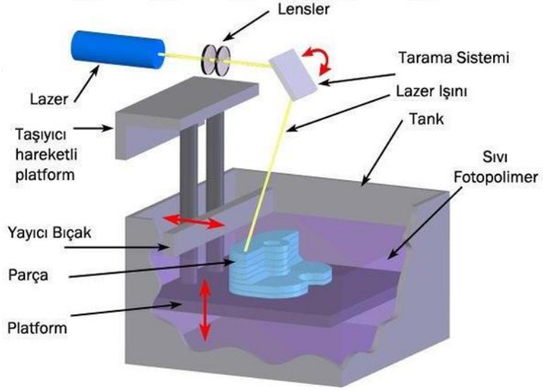
Resim 2 Katı Kütleme Teknolojisine Sahip 3D Yazıcı
