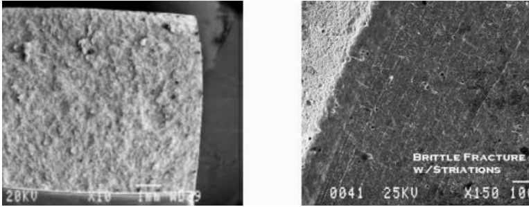
Şekil 2. Gevrek kırılma yüzeyinin SEM görüntüsü
