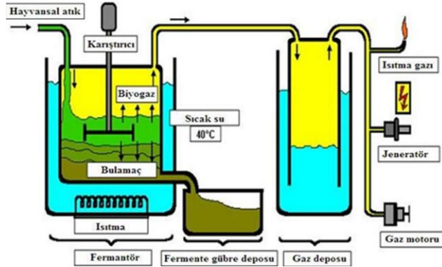
Şekil 1 Mikro biyolojik gaz prosesi
