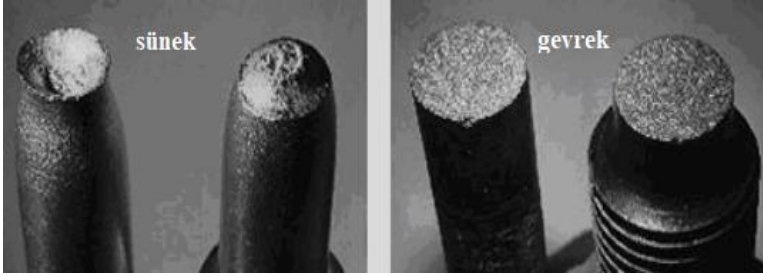
Şekil 4. Sünek ve Gevrek kırılma örneği
