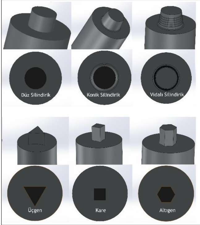
Şekil 5. SKNK da kullanılan uc profilleri
