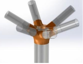
Resim 9 3D Yazıcı Teknolojisiyle Üretilmiş Çatı Kanopisi Bağlantı Elemanları
