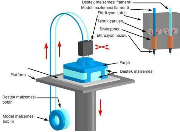
Resim 4 Eriyik Yığarak Modelleme Teknolojisine Sahip 3D Yazıcı
