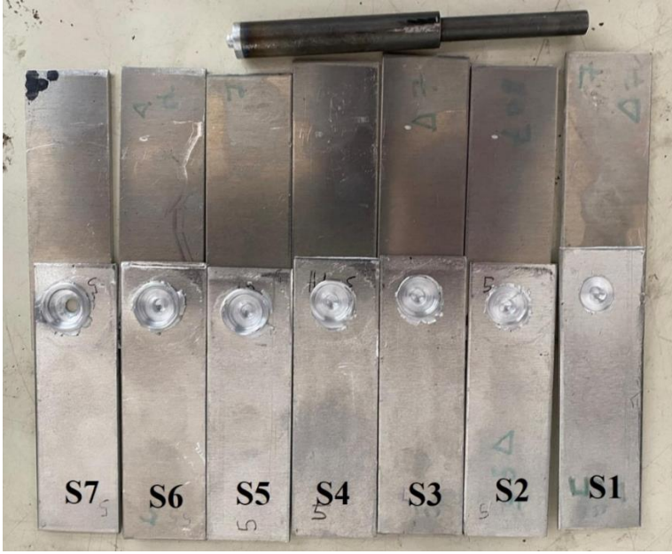
Şekil 6. SKNK ile birleştirilen farklı 7075 ve 5754 alüminyum alaşımları
