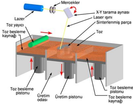
Resim 6 Seçmeli Lazer Sinterleme ve Ergitme Teknolojisine Sahip 3D Yazıcı
