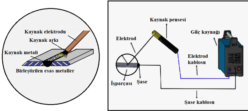
Şekil 1. Elektrik ark kaynağının şematik resmi
