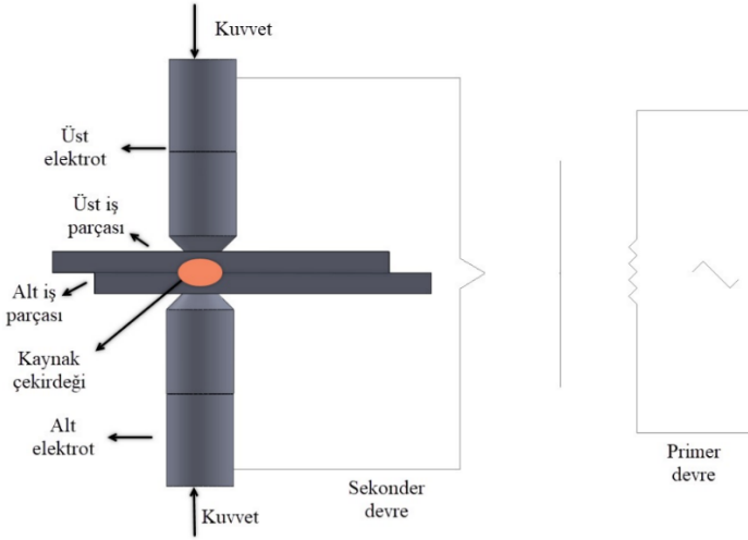
Şekil 3. Nokta direnç kaynağının şematik resmi
