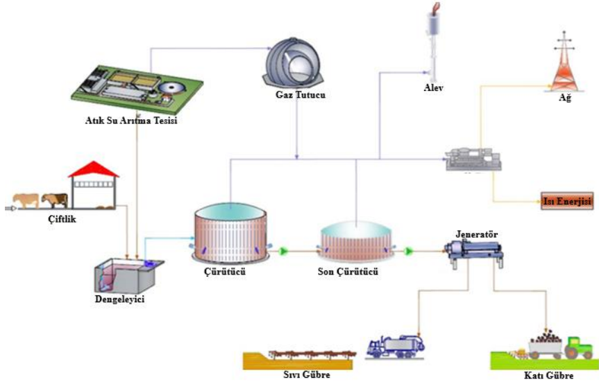
Şekil 2 Makro biyolojik gaz prosesi
