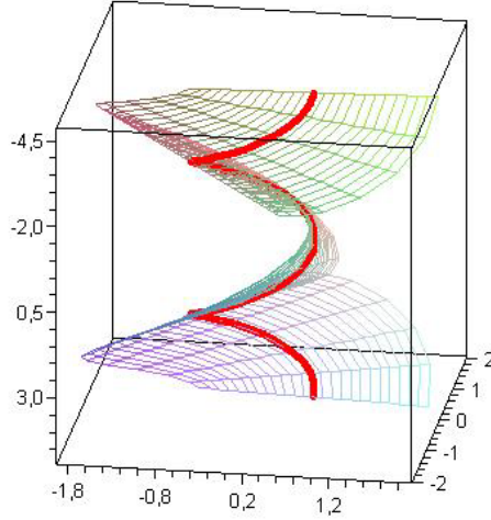
Şekil 8 \delta eğrilik çizgili yüzey ailesinin bir üyesi
