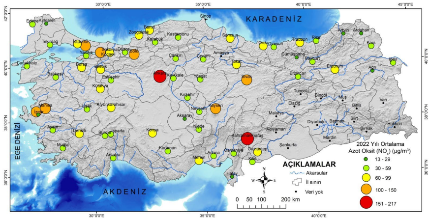
Şekil 8: Türkiye’de Yıllık Ortalama Azot Oksit(NO x ) Konsantrasyonlarının Dağılışı (2022)
