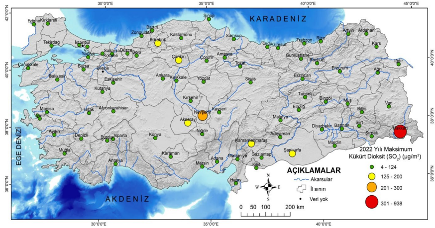
Şekil 2: Türkiye’de Maksimum Kükürt Dioksit ( \text{SO}_2 ) Konsantrasyonlarının ( \mu\text{g}/\text{m}^3 ) Dağılışı (2022)
