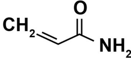
řekil 1 Akrilamid kimyasal yapısı
