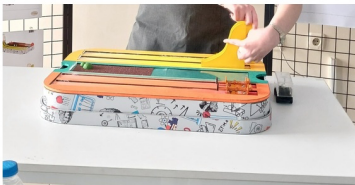
Şekil 4. Fiziksel işlem önerilerinin prototiplere yansımaları: (A) hareket hatları, (B) bağlantı/kurulum tablosu.
