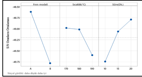
Şekil 7. Ana etkenler ile elde edilen kek ağırlığının S/N oranlarının ortalama grafiği
