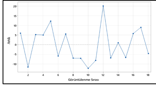
Şekil 15. Kek ağırlığı için regresyon kalıntılar görüntülenmek sırasına karşı grafiği
