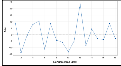
Şekil 10. Kek ağırlığı için ANOVA kalıntılar görüntülenmek sırasına karşı grafiği
