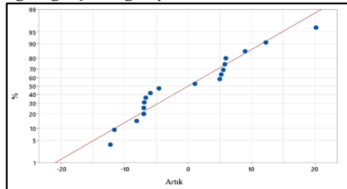
Şekil 11. Kek ağırlığı için regresyon analizinin normal olasılık grafiği
