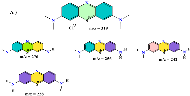
Şekil 6 a) CuO nanopartikülü ile MB b) ZnO/CQD nanopartikülü MB'leri ışık ile c) ZnO/Ag 2 O/rGO ZnO/Ag 2 O/rGO heteroyapılı katalizör ile karanlıkta bozunumu
