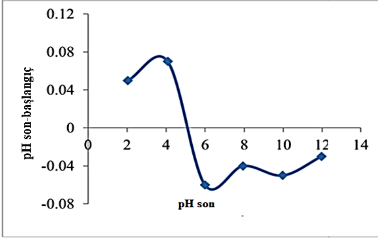
Şekil 2 ZST ait pcz grafiği
