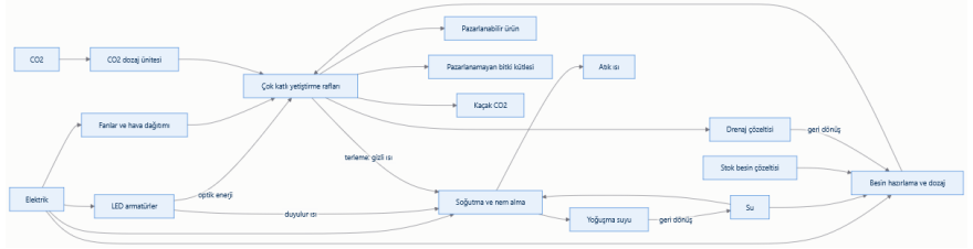
Şekil 1. Çok katlı kapalı bir üretim sisteminde enerji, su, CO 2 ve besin maddesi akışlarının şematik gösterimi
