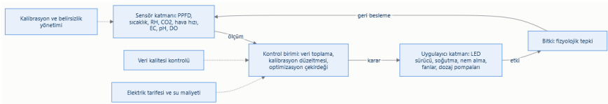
Şekil 4. Sensör–kontrol birimi–uygulayıcı–bitki geri besleme döngüsü
