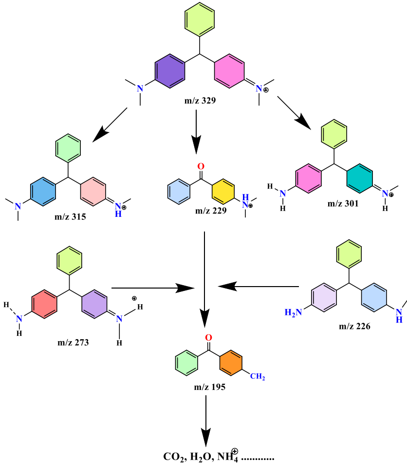
Şekil 5 MG boyasının ZnO NP leri varlığında fotobozunumu sırasında oluşan ara ürünler
