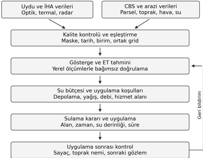
Şekil 1. Uzaktan algılama ve CBS ile sulama kararının oluşturulması
