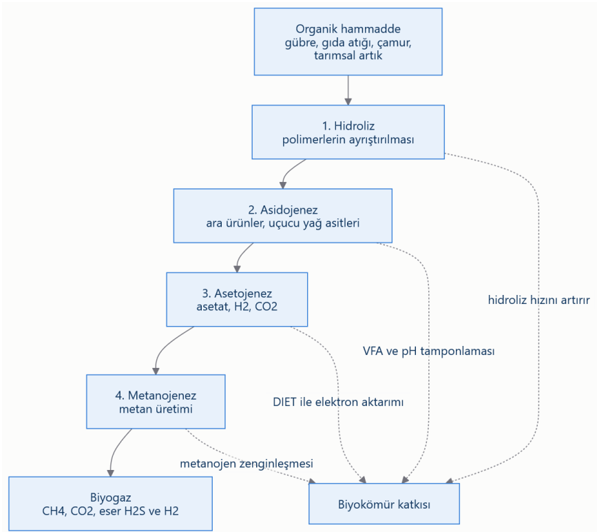
Şekil 1. Anaerobik çürütmenin dört aşamalı biyokimyasal dönüşümü ve biyokömürün müdahale ettiği süreç noktaları
