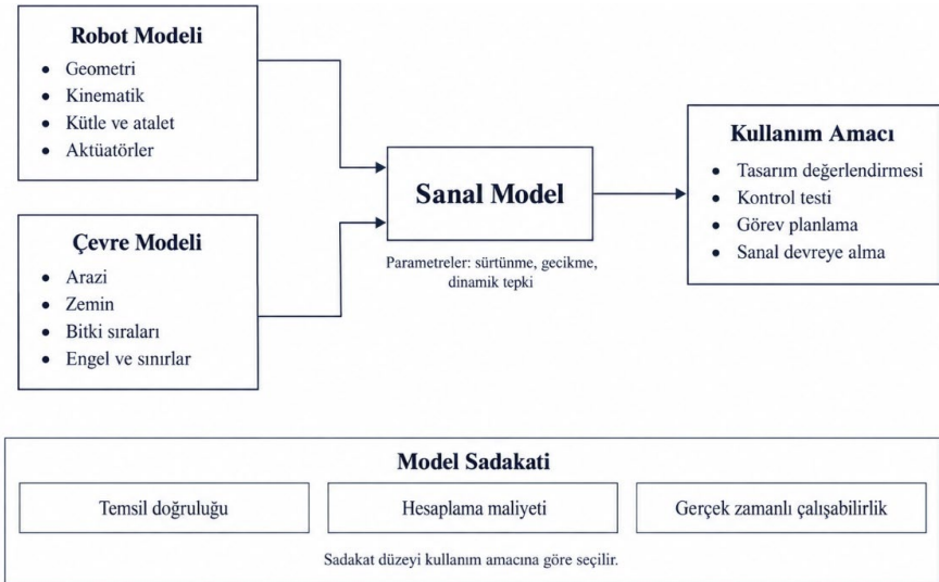
Şekil 2 Tarımsal mobil robotlarda sanal model ve model sadakati
