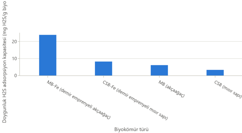
Şekil 5. Demir emprenyeli ve modifiye edilmemiş biyokömürlerin doygunluk H 2 S adsorpsiyon kapasitelerinin karşılaştırılması
