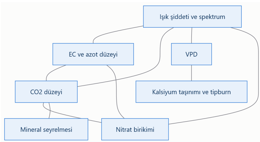
Şekil 4. Işık, mikroiklim ve bitki beslemesi arasındaki başlıca etkileşimler ve kalite üzerindeki hedef değişkenler.
