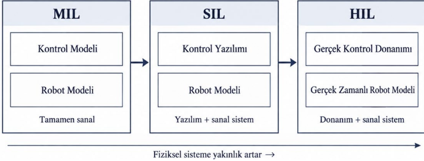
Şekil 3 MIL–SIL–HIL tabanlı sanal devreye alma süreci
