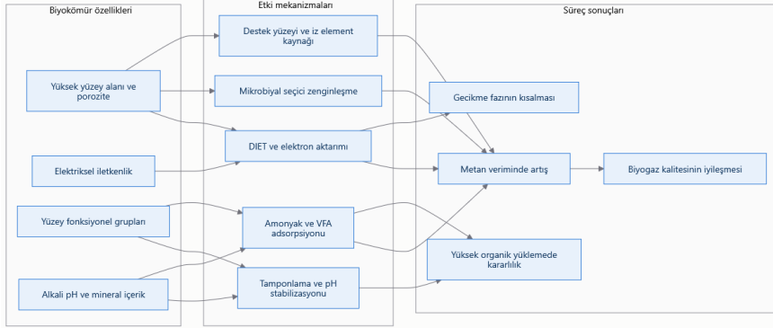
Şekil 3. Biyokömürün fizikokimyasal özellikleri, etki mekanizmaları ve anaerobik çürütme performansı arasındaki ilişki ağı
