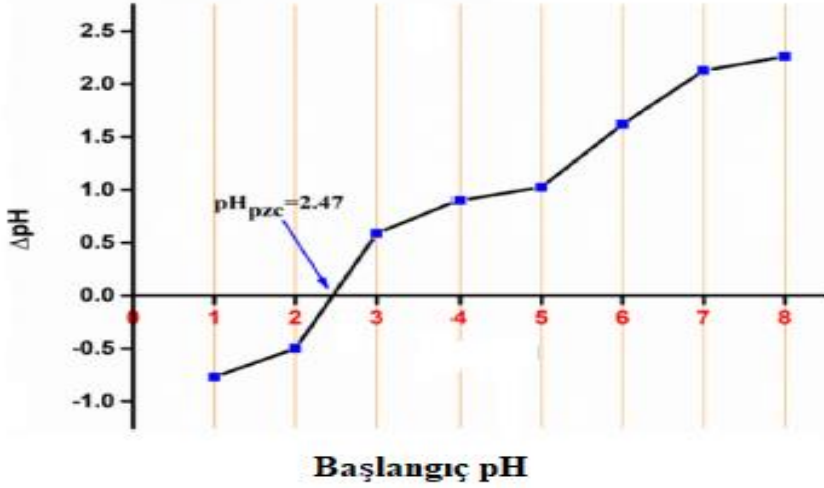
Şekil 1 N-C-dots/SgCN/gCN yapısının pH pzc değerinin gösterimi
