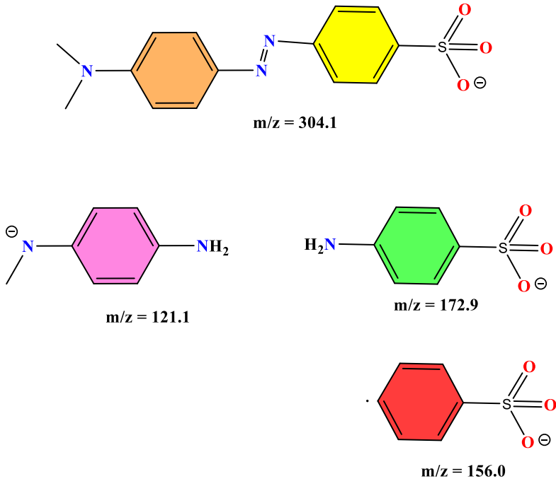
Şekil 4 ESI/MS temelinde MO boyar maddesine ait ana ara ürünlerin önerilen yapıları
