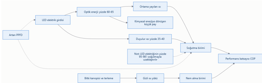
Şekil 2. Aydınlatma ile soğutma ve nem alma yükleri arasındaki ilişkiyi açıklayan kavramsal şema
