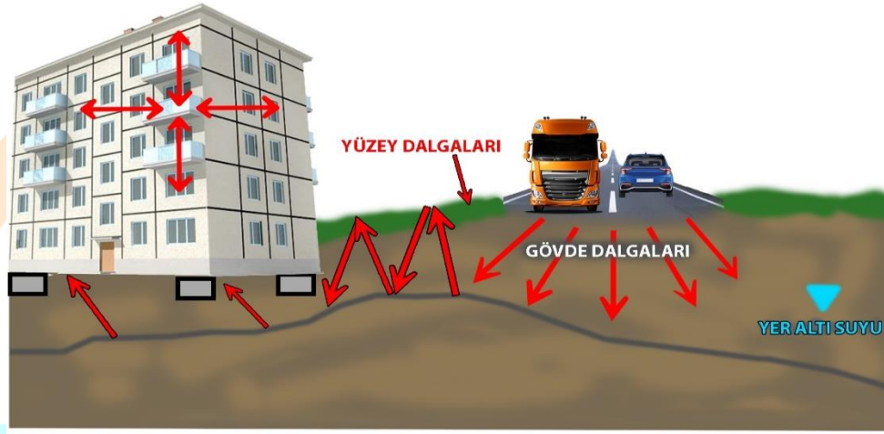
Şekil 1. Karayolu titreşiminin yayılımı
