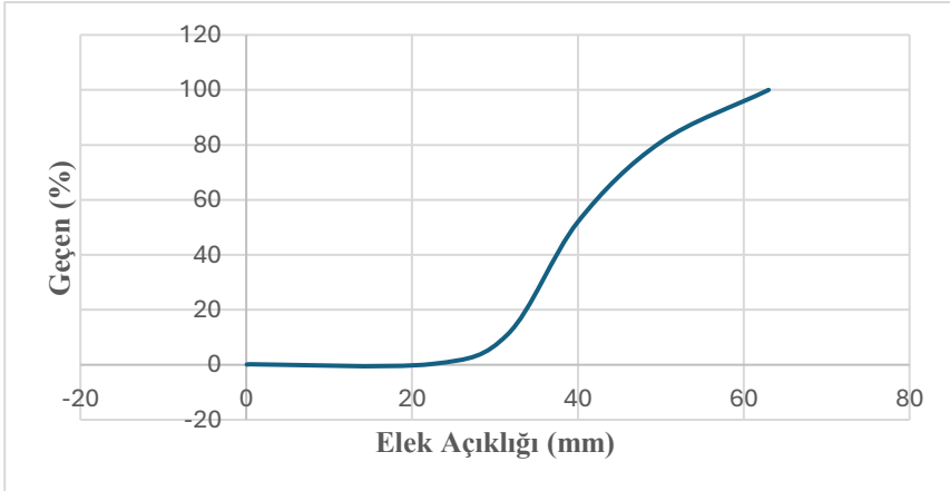
Şekil 6. Işıkkara (Kütahya) kırma bazalt agregaların Tane boyu dağılım grafiği
