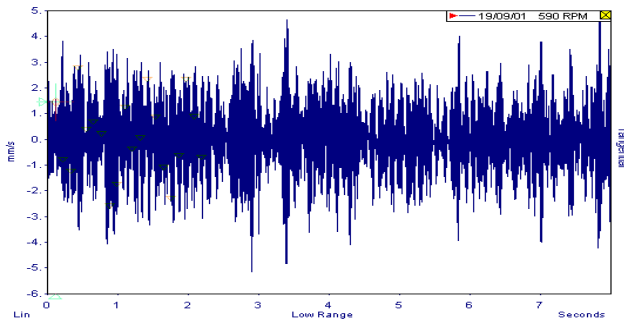
Şekil 34. Şaft rulman yatağı tanjantiyal yön dalgaformu grafiği
