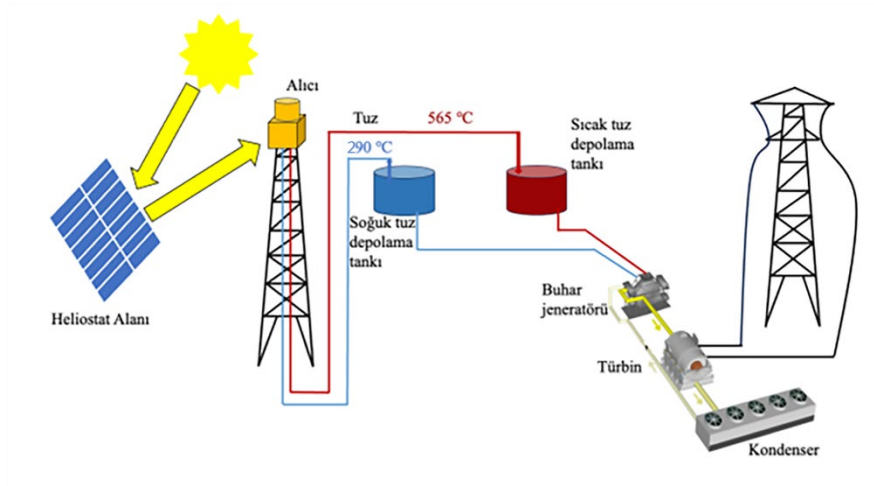
Resim 2 Güneş kulesi santralının şematik diyagramı
