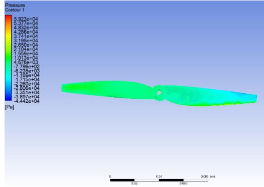
Şekil 10. Basınç analizi kontur dağılımı
