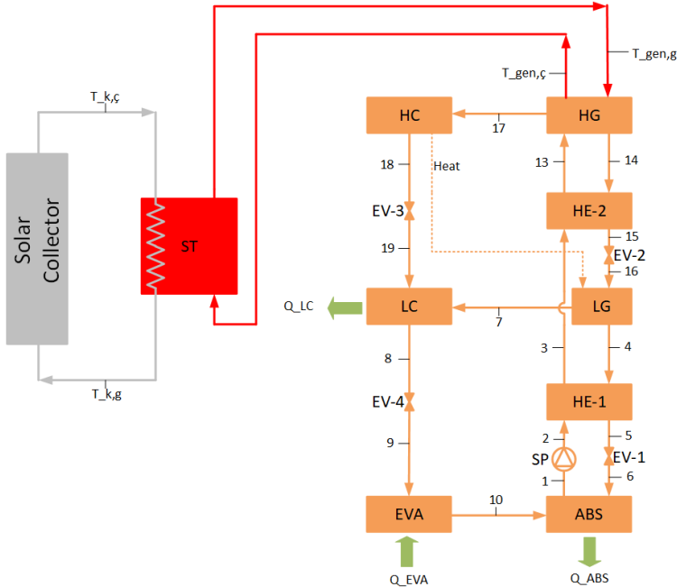
Şekil 1 Çift kademeli güneş enerjili absorpsiyonlu soğutma sistemi
