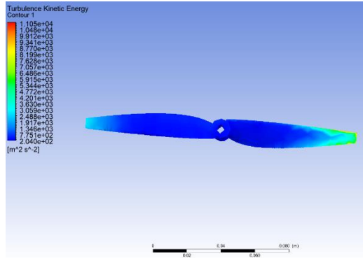
Şekil 7. Turbulence Kinetic Energy analiz sonuçları
