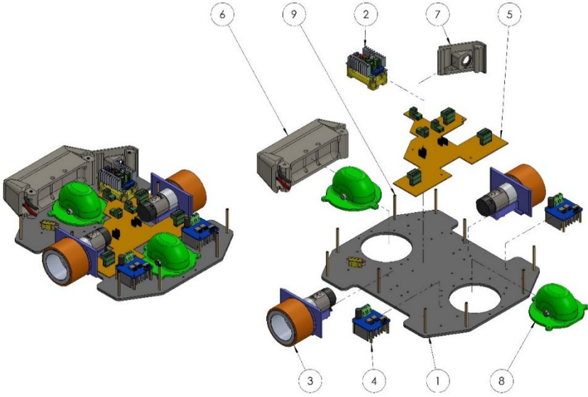
Şekil-2. Robot Mekanik Komponentleri
