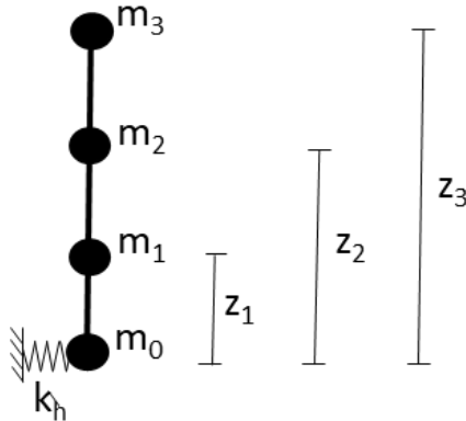
Şekil 4 Temel kütleli ÇSD'li sistem
