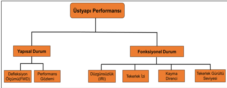
Şekil 3 Üstyapı Yapısal ve Fonksiyonel Durum Tespit Yöntemleri
