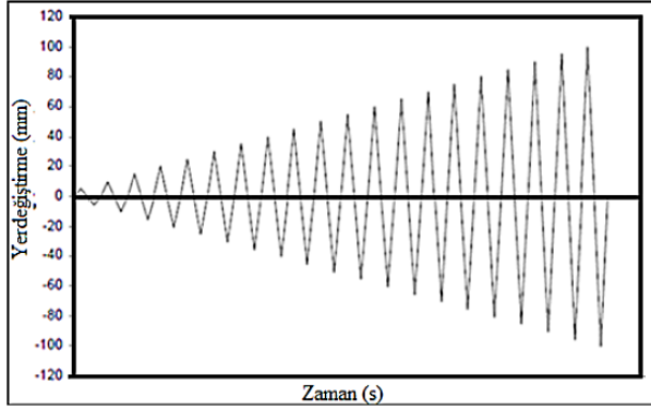
Şekil 5 Deneylerde uygulanan yer değiştirme
