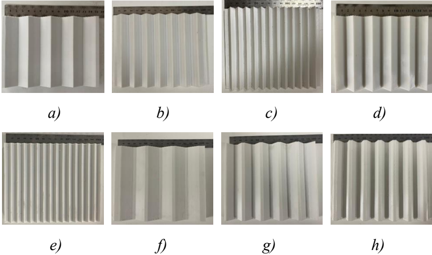
Şekil 6. Basılan prototip istinat tabanı pürüzleri a) Prototip-1, b) Prototip-2b, c) Prototip-3, d) Prototip-2c, e) Prototip-2a, f) Prototip-4, g) Prototip-5, h) Prototip-6
