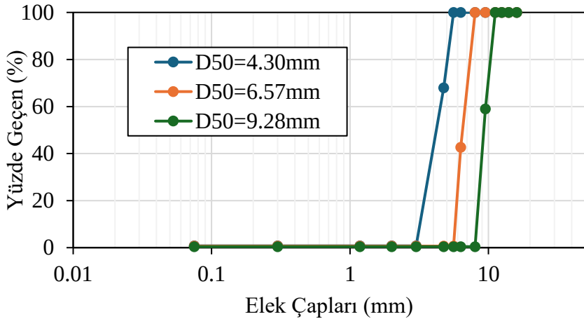
Şekil 2 Zeminlerin gradasyonları
