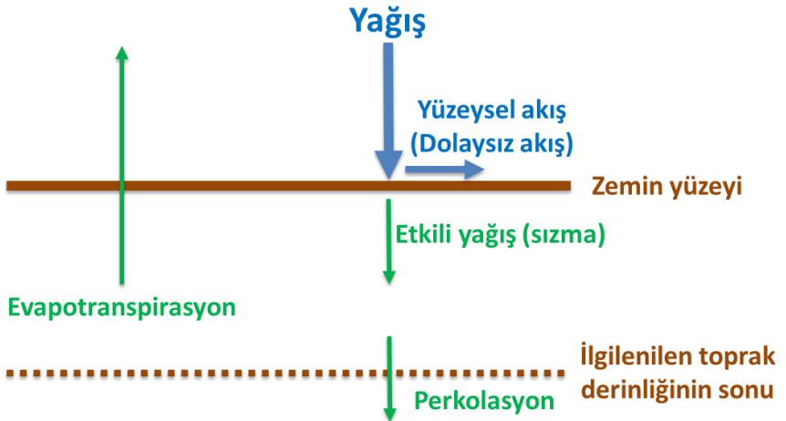
Şekil 4 Hidrolojik modelin temel şeması.
