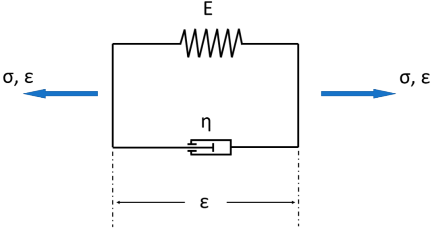
Şekil 2. Viskoelastik davranışı tanımlamak için yay ve sönümleyiciden oluşan basit bir model. (Kelvin–Voigt model). Modelde E =Elastikiyet modülü, \epsilon = strain, \eta = viskosite, \sigma = gerilim (stress) değerlerini ifade etmektedir (Eschweiler ve ark., 2021).
