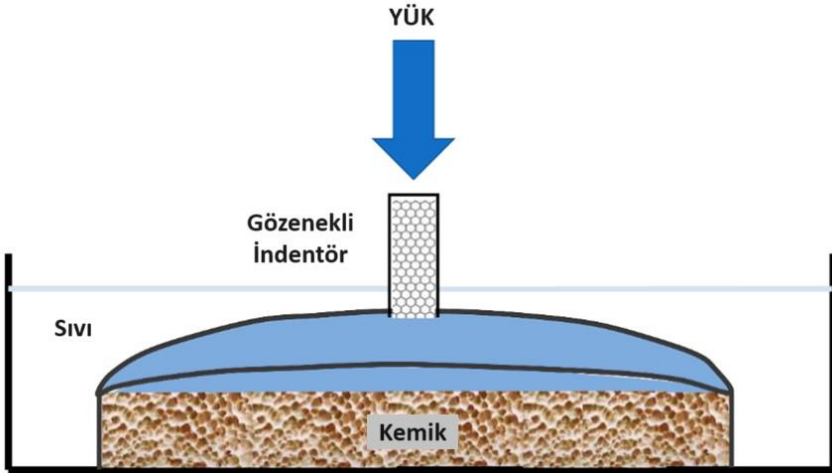
Şekil 7. Eklem kıkırdağı üzerinde bir girinti testi gerçekleřtirmek için kullanılan bir aparatın temsili (Huyghe ve ark., 1997).
