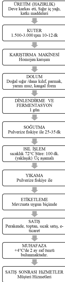
Şekil 2.4. Modern Yöntemle (Isıl İşlem) Üretilen İncirlioiva Deve Sucuğunun Üretim Akış Şeması
