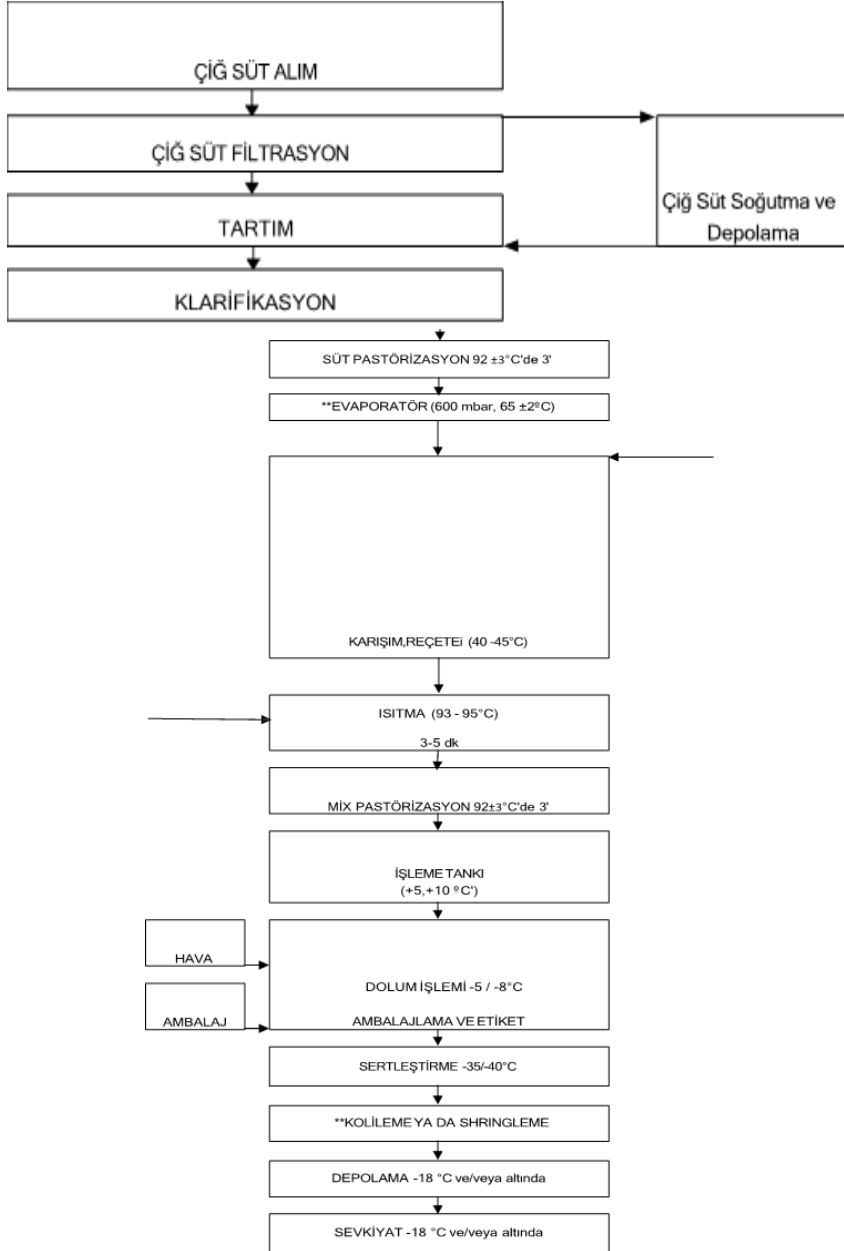
Şekil 1.1: Maraş dondurması üretim akış şeması
