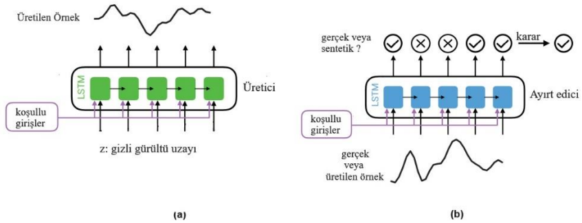
Şekil 13. (a)Tekrarlayan GAN (RGAN) ve (b)Tekrarlayan Koşullu GAN (RCGAN) mimarileri (Esteban, Hyland & Rätsch, 2017)
