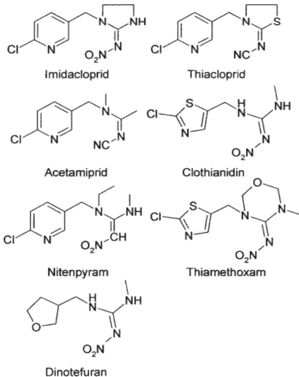
Şekil 1. Neonikotinoid insektisitlerin kimyasal yapıları (Nauen, & Denholm, 2005).
