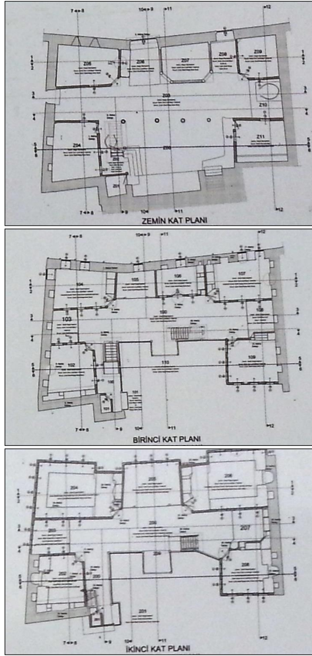
Şekil 4.3. Çakırağa Konağı Kat Planları
