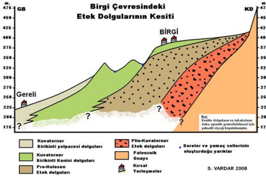
Şekil 4.1. Birgi ve Çevresindeki Etek Dolgularının Kesiti
