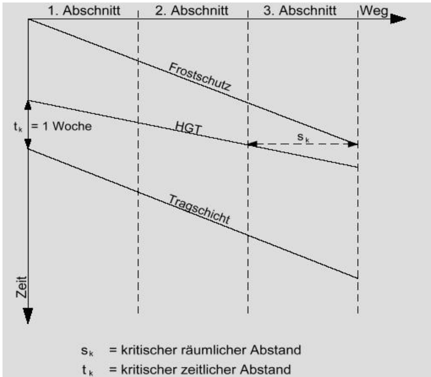
Abbildung 8: Beispiel Zeit-Wege Diagramm
