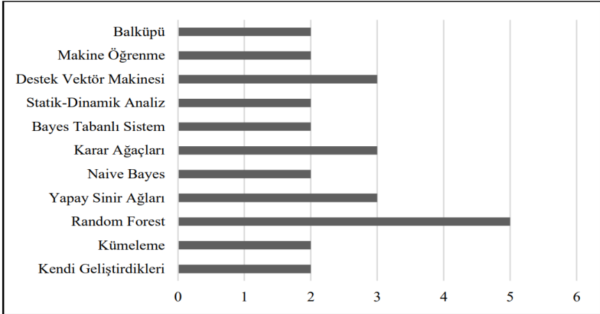
Şekil 17. En çok kullanılan saldırı tespit yöntemleri (Hatipoğlu ve Tunacan, 2021: 12).
