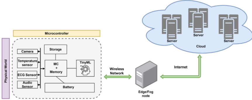
Şekil 2. TinyML'in IoT iş akışına entegrasyonunu
