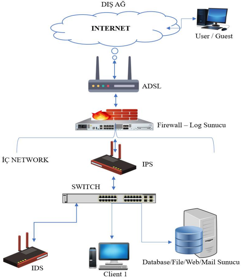
Şekil 20. Saldırı önleme sistemi IDS/IPS.
